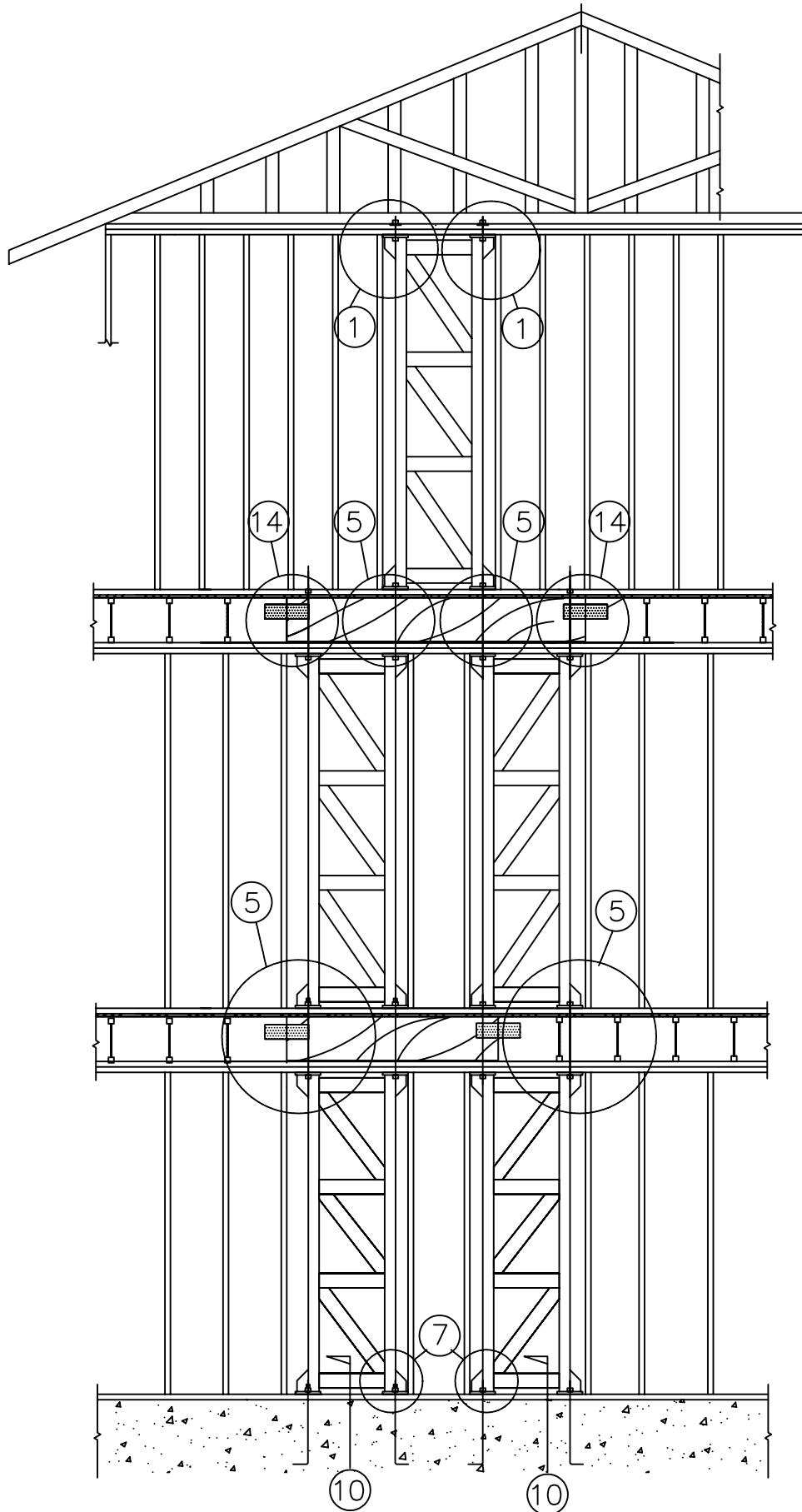
PYRAMID 1-2-2 SCALE: N.T.S.
