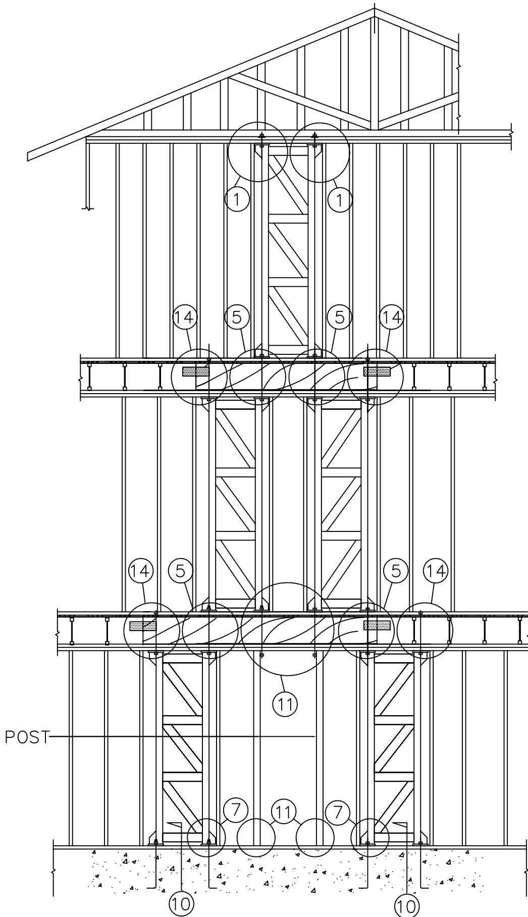
PYRAMID 1-2-2 W/POSTS SCALE: N.T.S.
