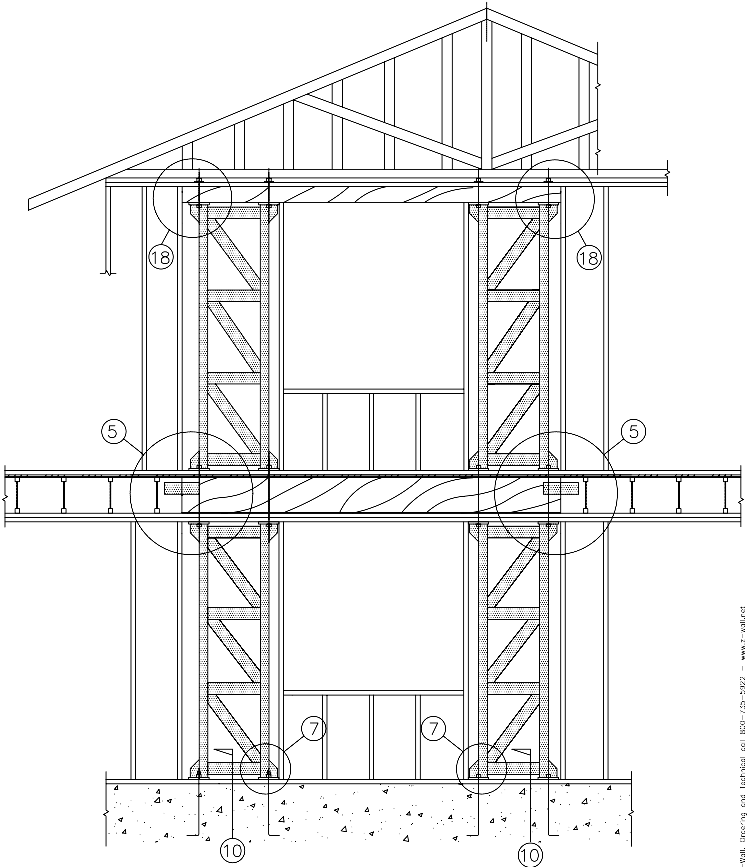
TWO STORY STACK SCALE: N.T.S.
