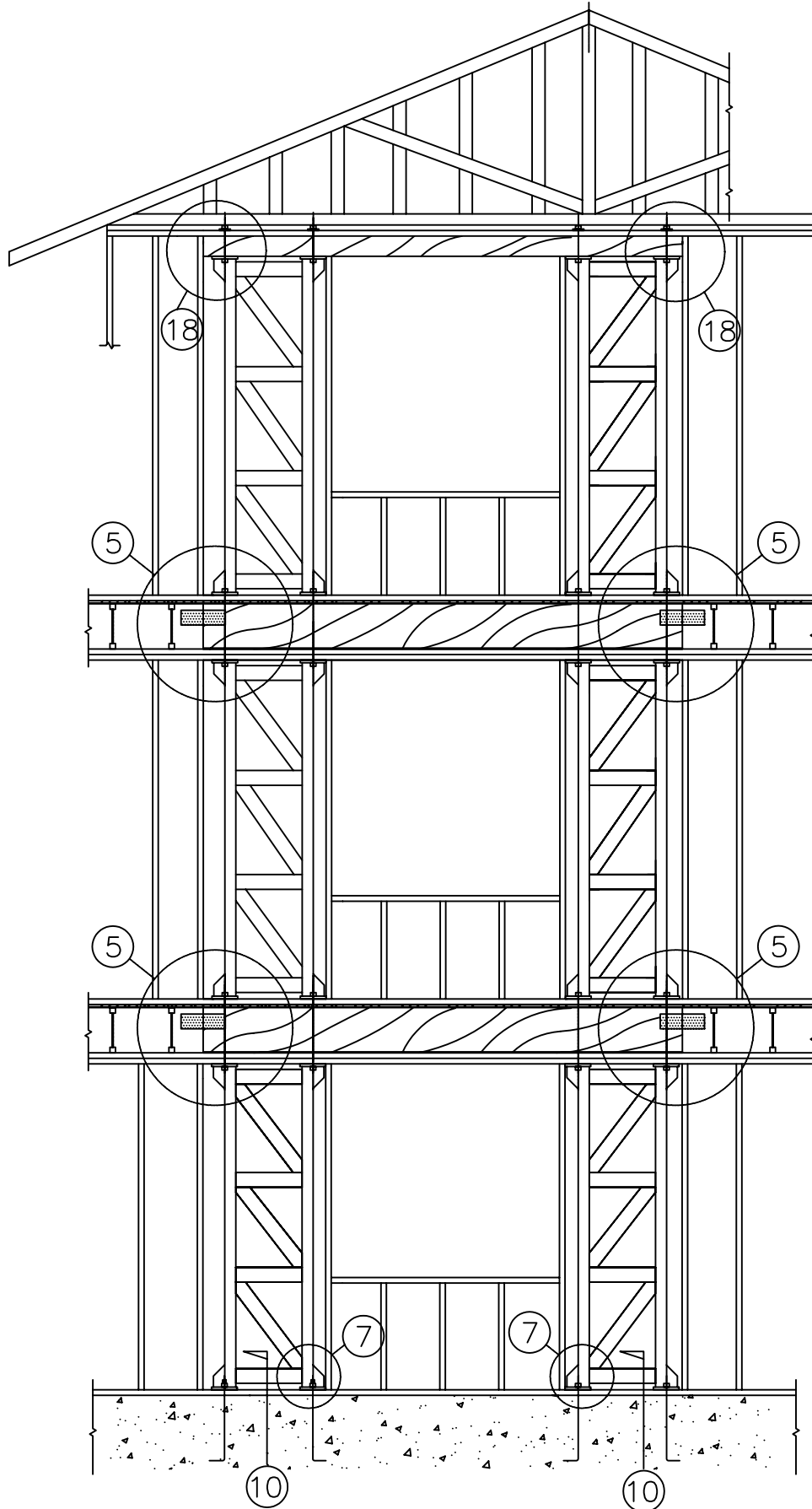
STACK 2-2-2 SCALE: N.T.S.
