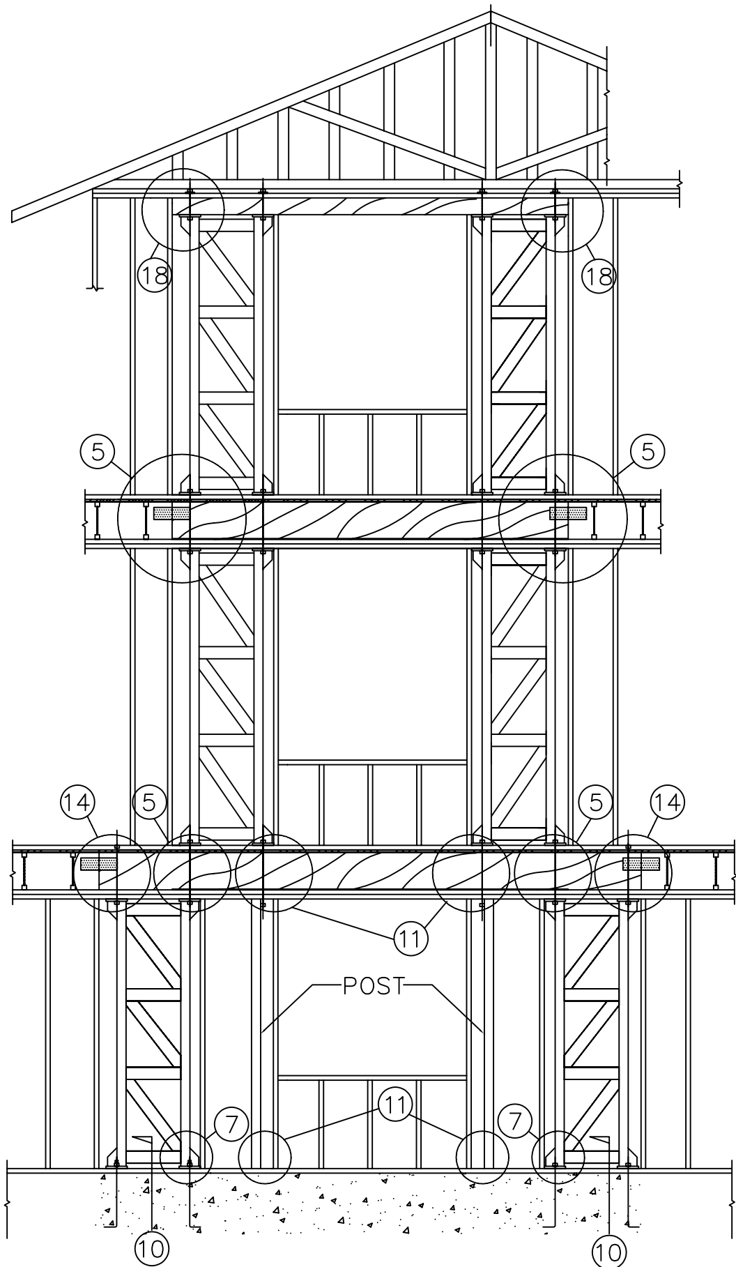
PYRAMID 2-2-2 W/POSTS SCALE: N.T.S.
