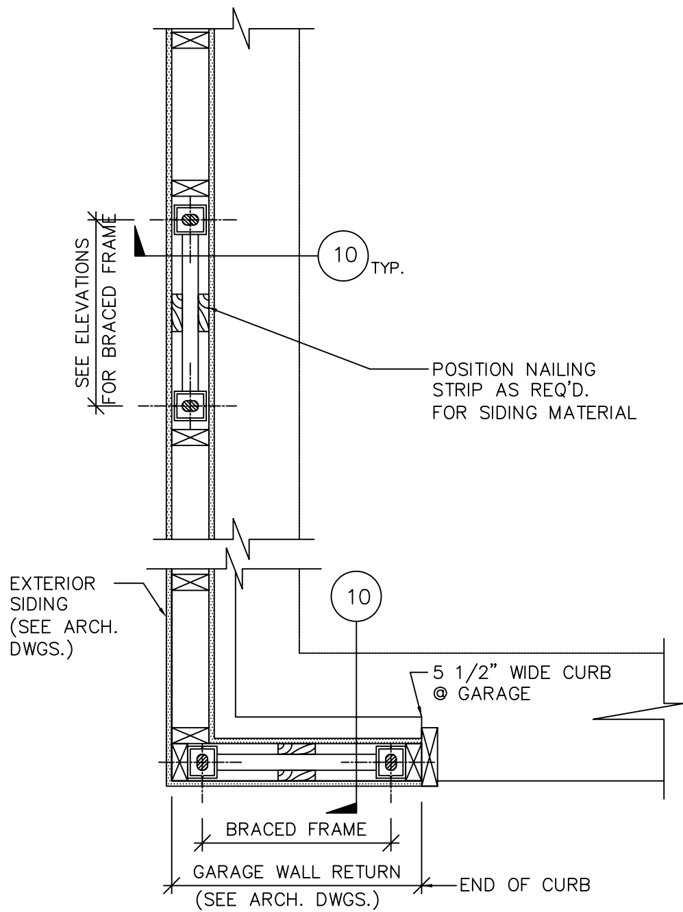
8 PLAN DETAIL N.T.S.
